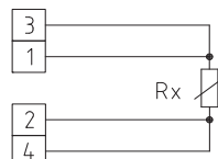
1x Vierleiterschaltung
